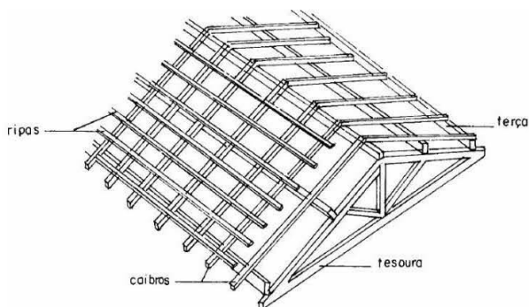
Figura 12: Ilustração de nomenclatura de elementos de estrutura de madeira do telhado.
